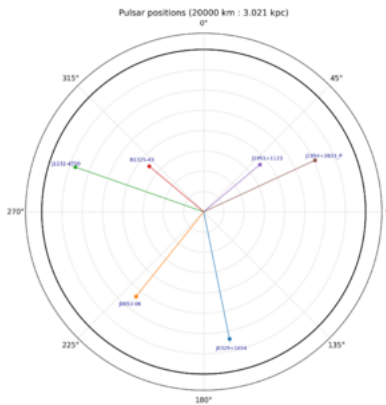
图f2 II 脉冲星地图
